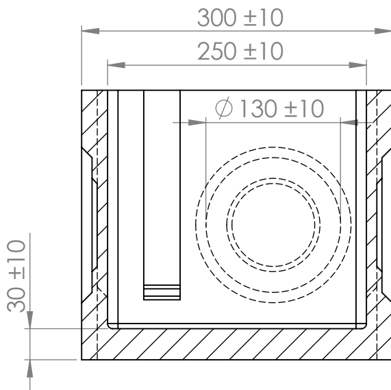
Prerez 2-2
