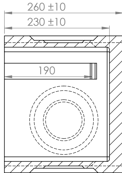
Prerez 1-1
